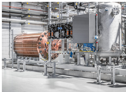
Power-to-Gas-Anlage in Grenzach-Wyhlen (Bild: Energiedienst / Daniel Infanger)
