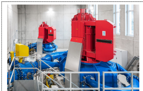
Turbinenhalle Wasserkraftwerk Gere im Wallis (Copyright: Troyer AG; Foto: www.meraner-hauser.com )
